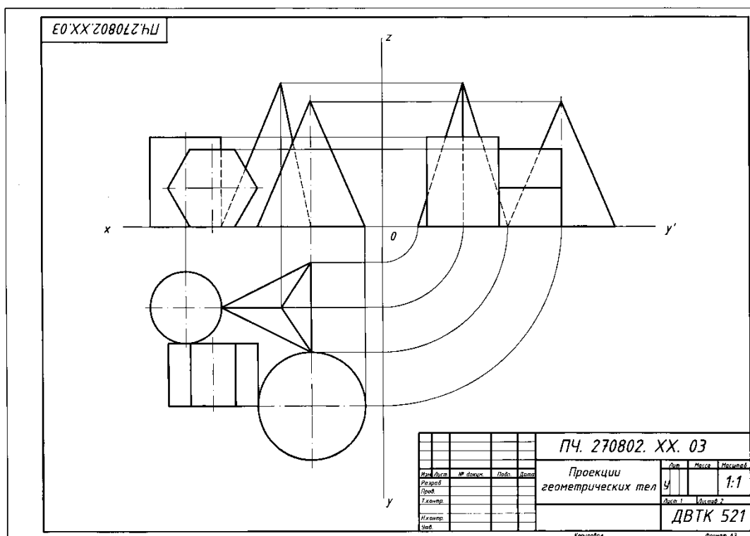
Рисунок 2.2.1 Пример выполнения графической работы № 4 а)
