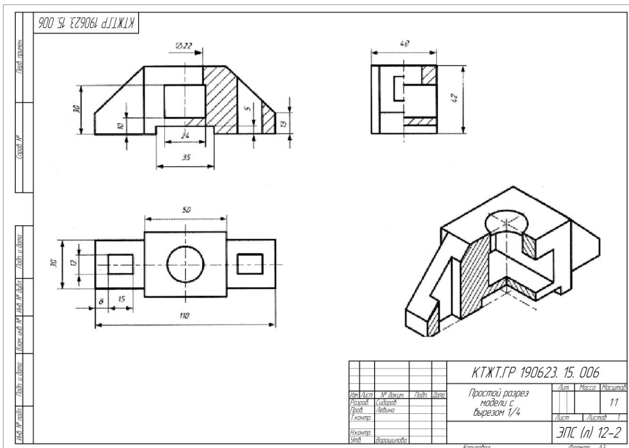
Рис. 4.2.6. Пример выполнения практической работы.
