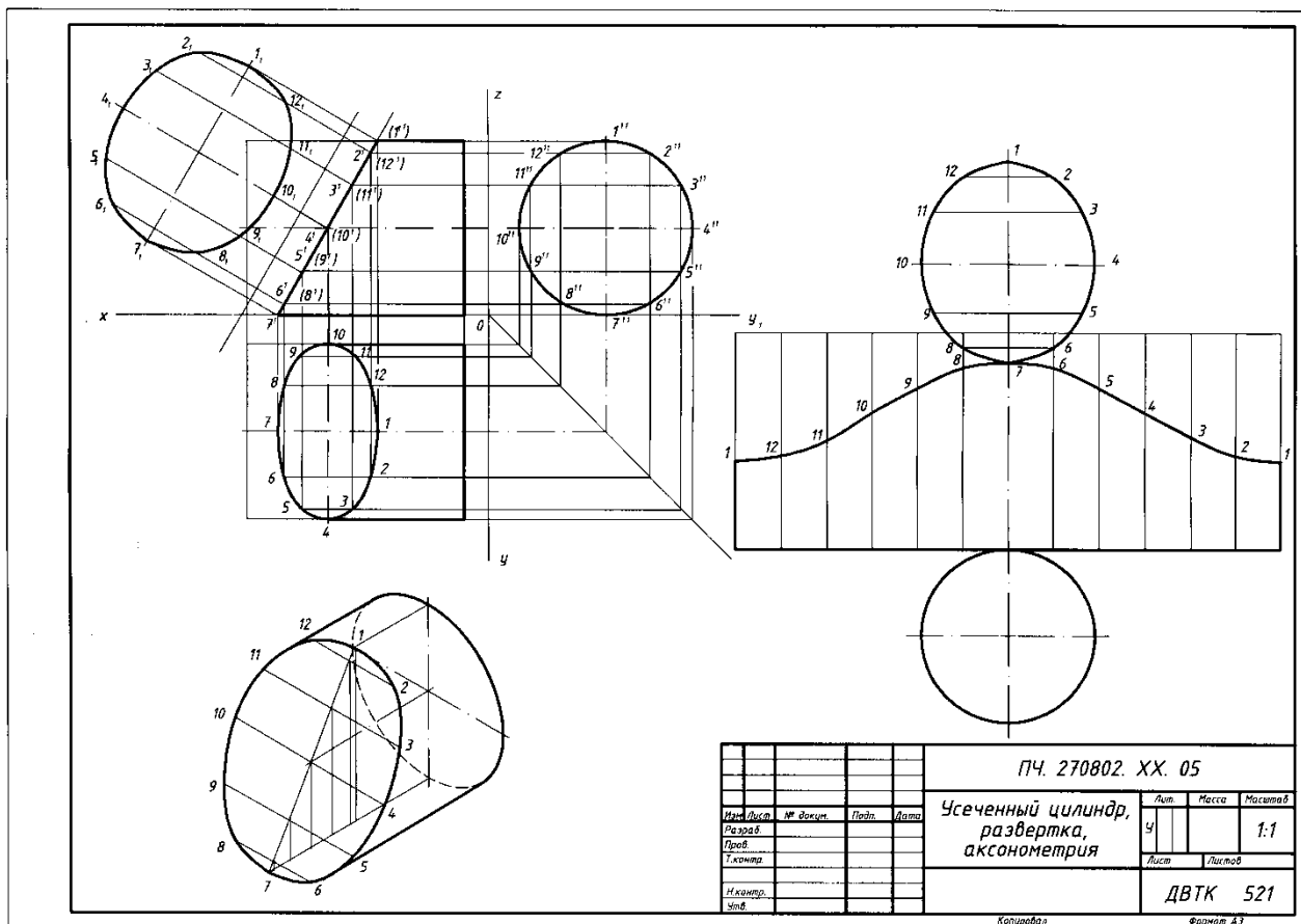
Рисунок 2.4.2. Пример выполнения графической работы № 6
