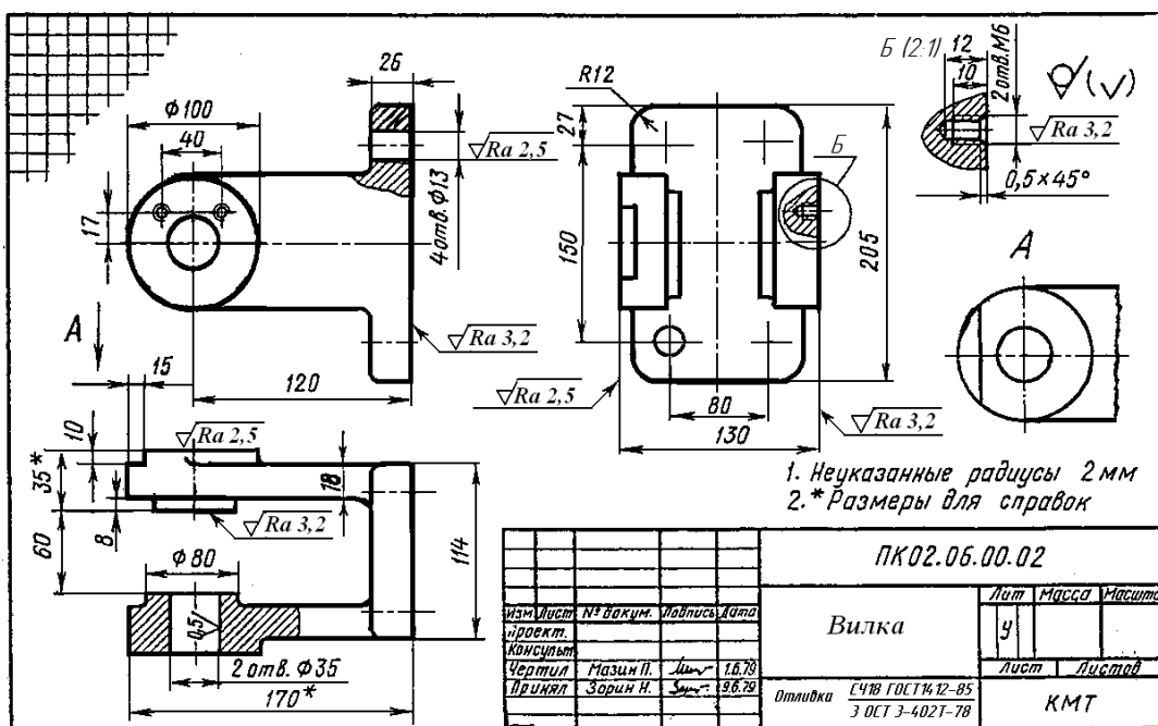
Рис. 4.3.4. Пример выполнения графической работы №15.
