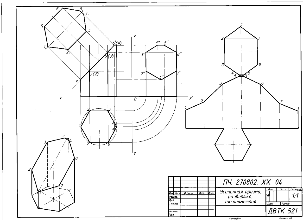
Рисунок 2.4.1. Пример выполнения графической работы № 5
