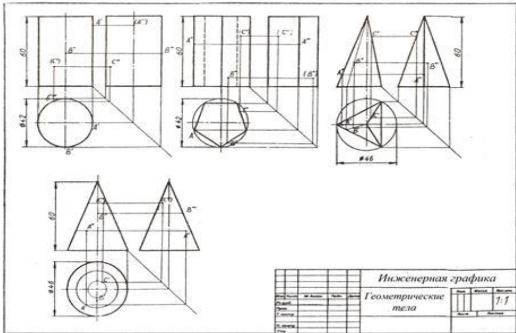
Рисунок 2.2.1 Пример выполнения графической работы № 3
