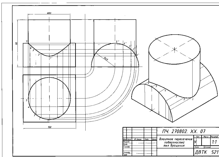
Рисунок 2.4.5. Пример выполнения графической работы №8 ЗАДАНИЕ К ГРАФИЧЕСКОЙ РАБОТЕ № 8
