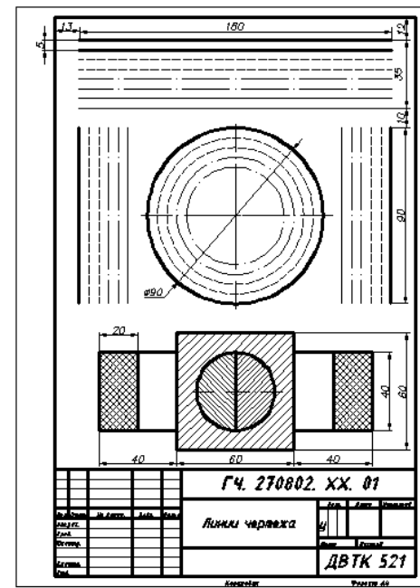
Рисунок 1.2.3. Пример выполнения графической работы № 1
