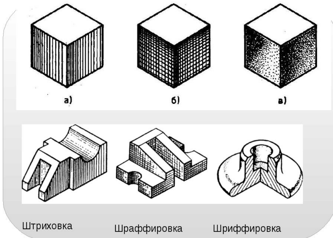
Рис. 3.1.1. Пример выполнения упражнений по выполнению технического рисунка.
