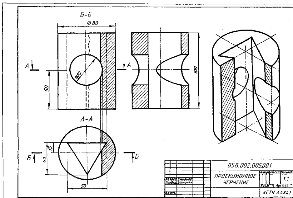
Рисунок 2.4.6 Пример выполнения практической работы №1
