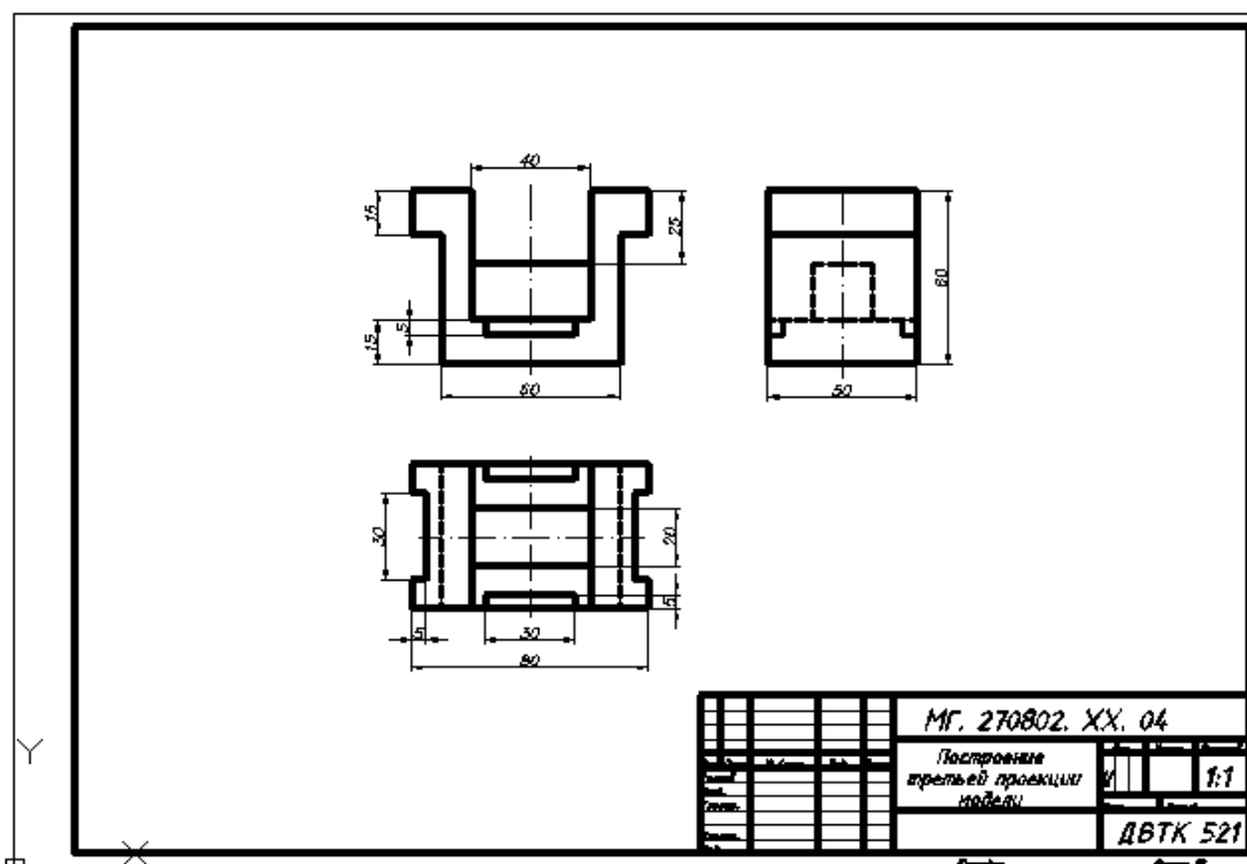
Рисунок 2.4.7. Пример выполнения графической работы № 9.
