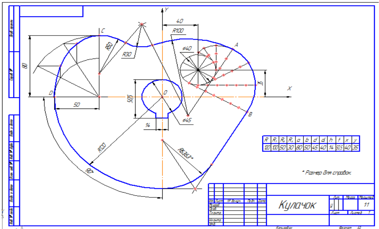
Рис.1.3.2. Пример выполнения практической работы №1.
