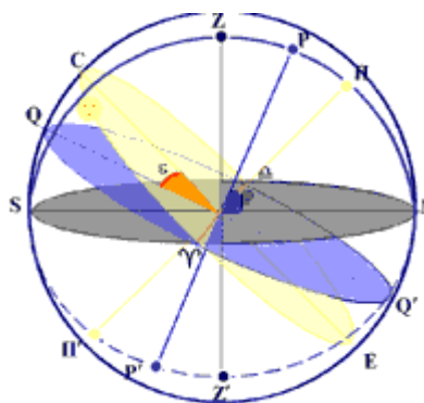
Рис.3 . Положение эклиптики на небесной сфере е точками весеннего (α) и осеннего (δ) равноденствий точками солнцестояний
